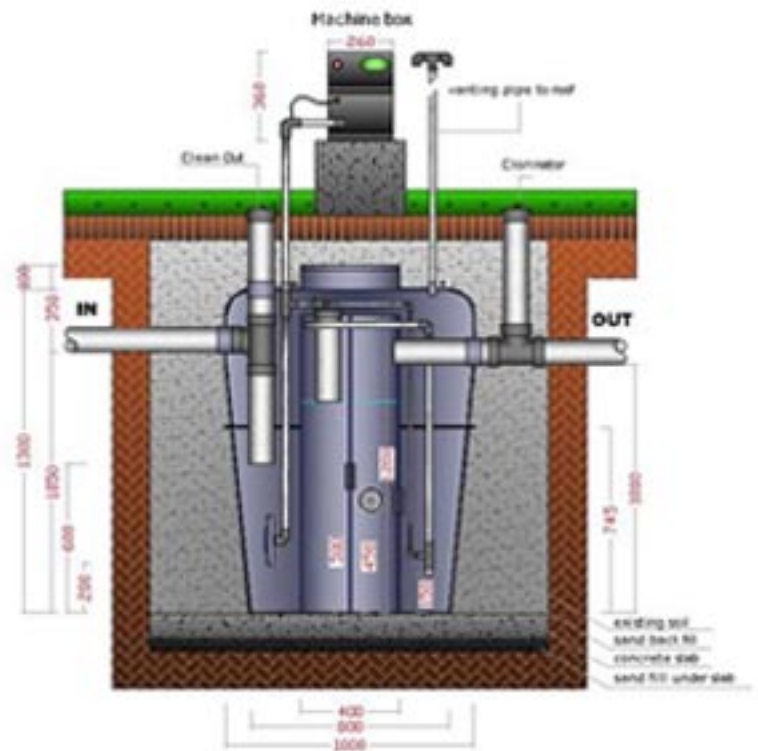
POTONGAN
